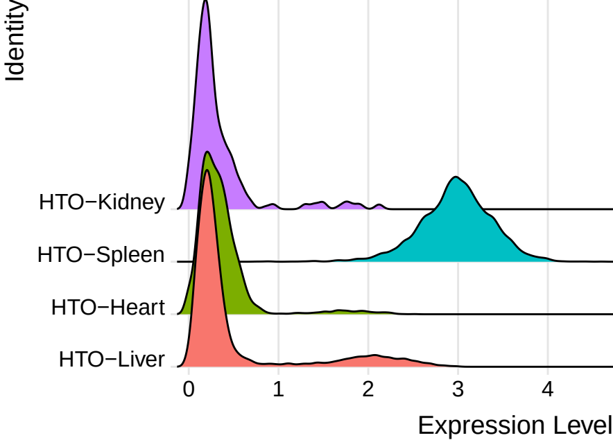
HTO-Spleen
