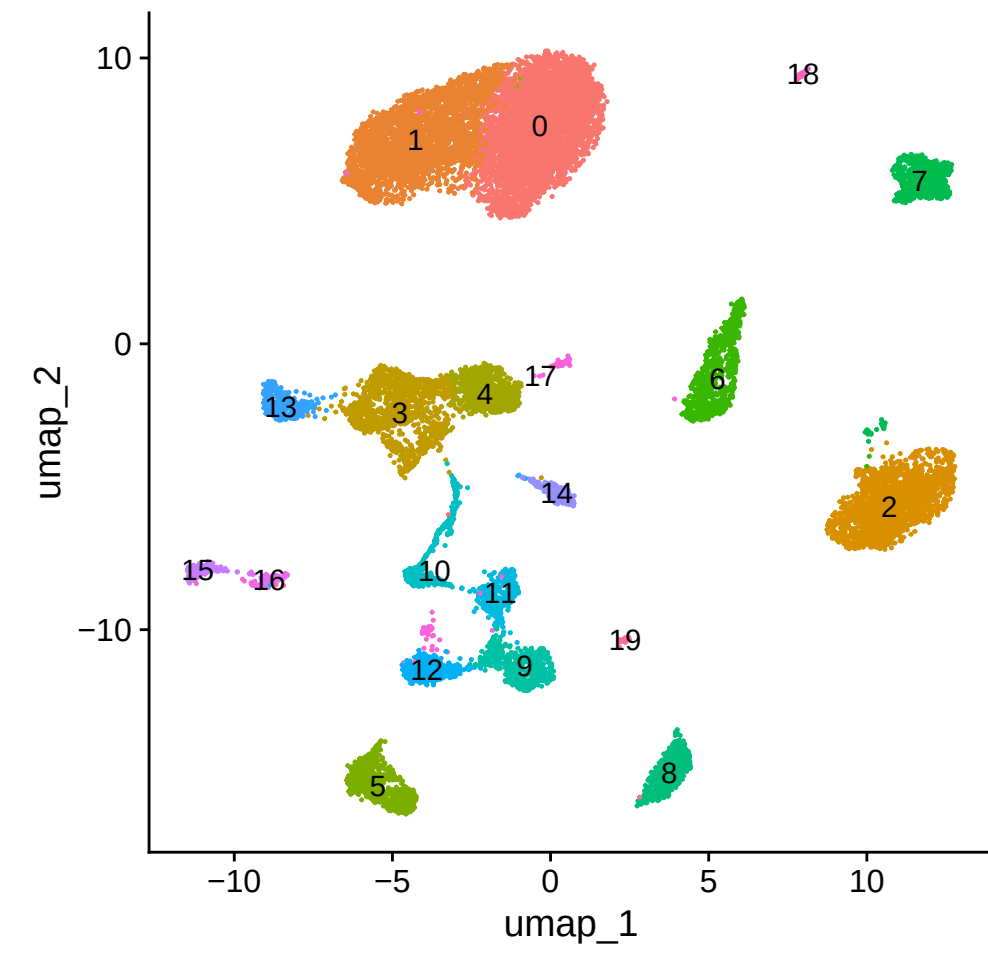
RNA_snn_res.0.6
