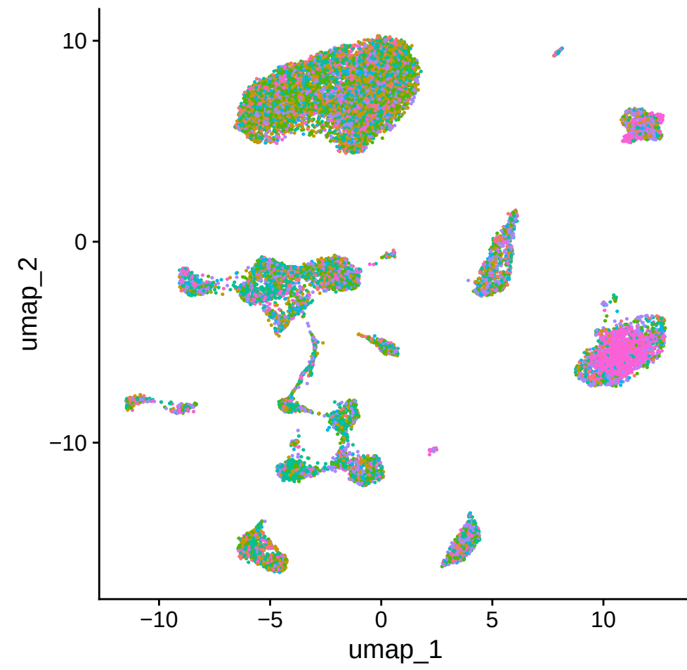
mouse_id
