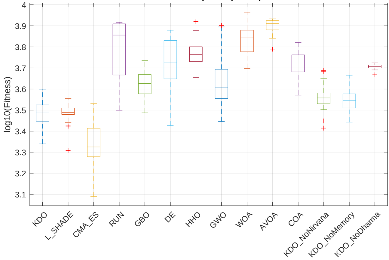
CEC2017 F10 (Partial) - Boxplot
