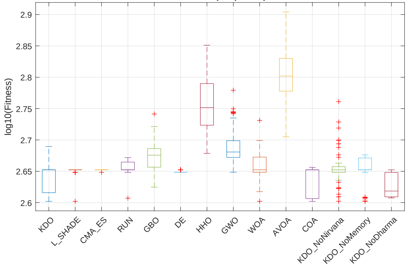
CEC2022 F2 (Full) - Boxplot
