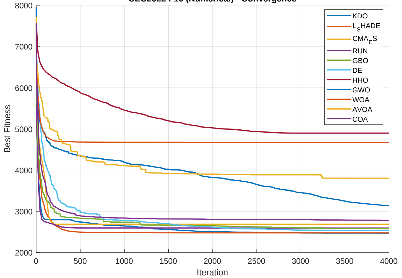
CEC2022 F10 (Numerical) - Convergence
