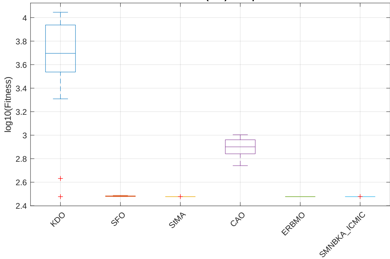
CEC2022 F1 (Full) - Boxplot
