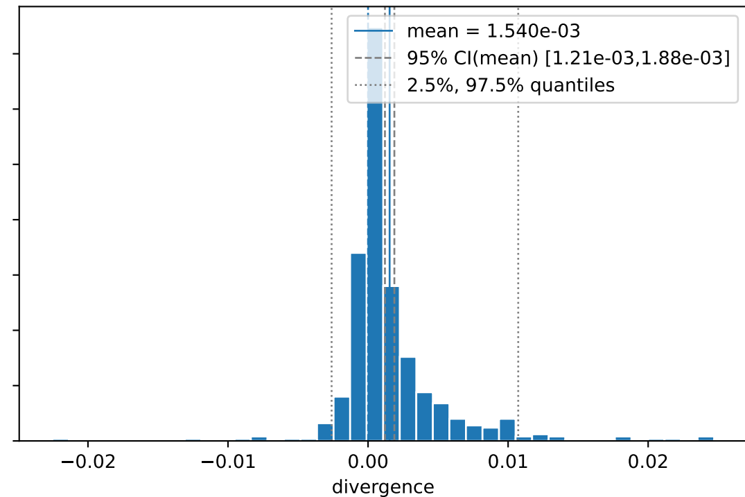
IPCW-oracle (n = 20000)
