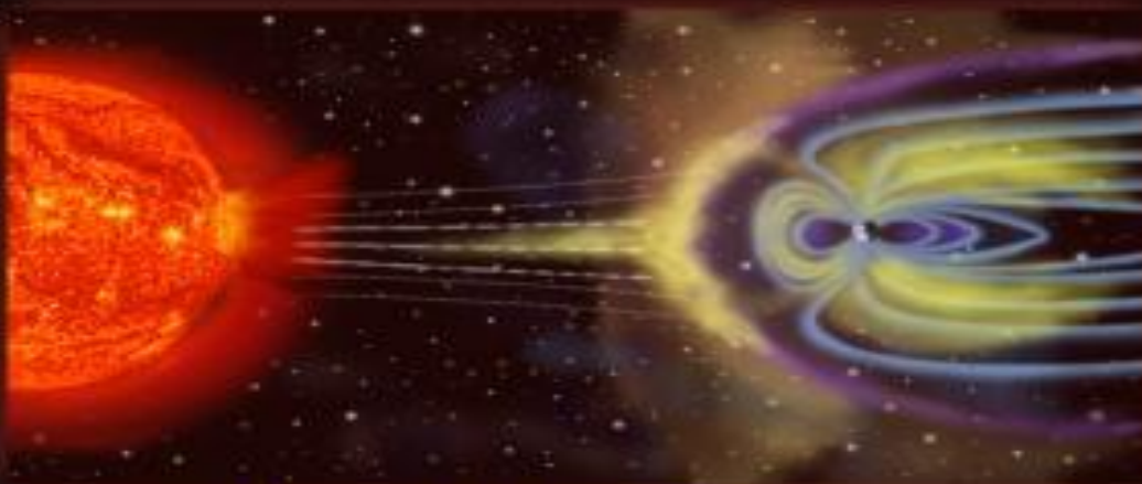
Magnetosfera Terrestre
