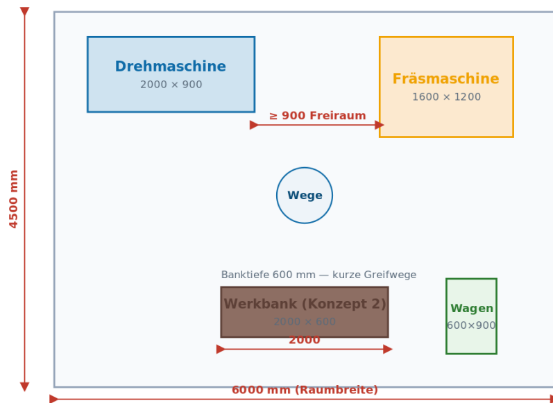
Abbildung 5.3: Maßstablicher Werkstatt-Grundriss
