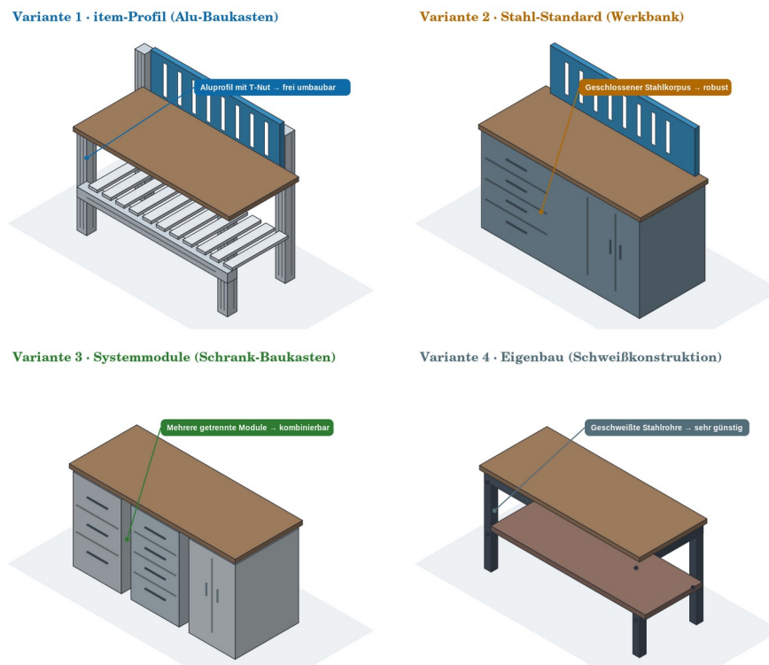
Abbildung 5.1: Vier untersuchte Bauvarianten der Werkbank im Vergleich
