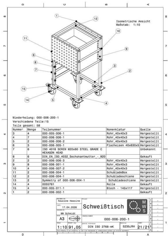
Abbildung 4.4: Zeichnungsblatt der Gesamtbaugruppe mit Stückliste
