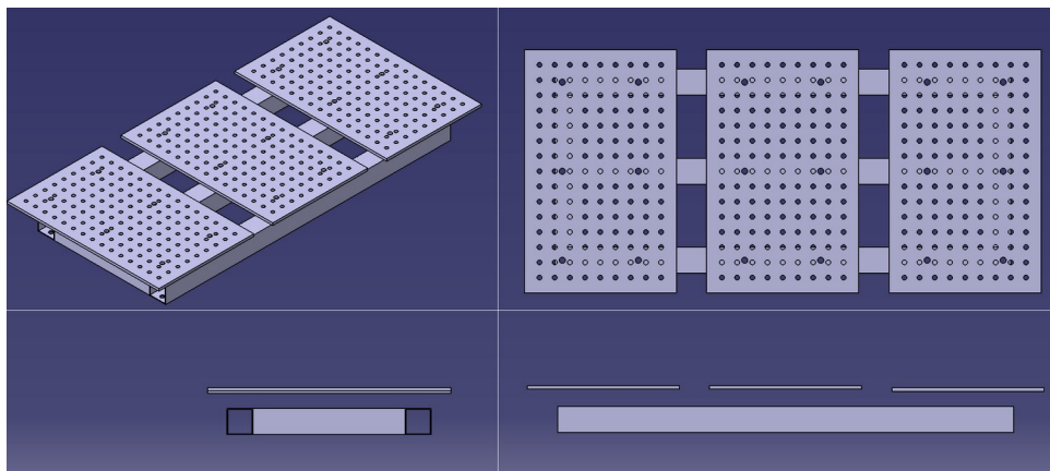
Abbildung 3.2: Lochplatten-Spannsystem auf dem Tischrahmen
