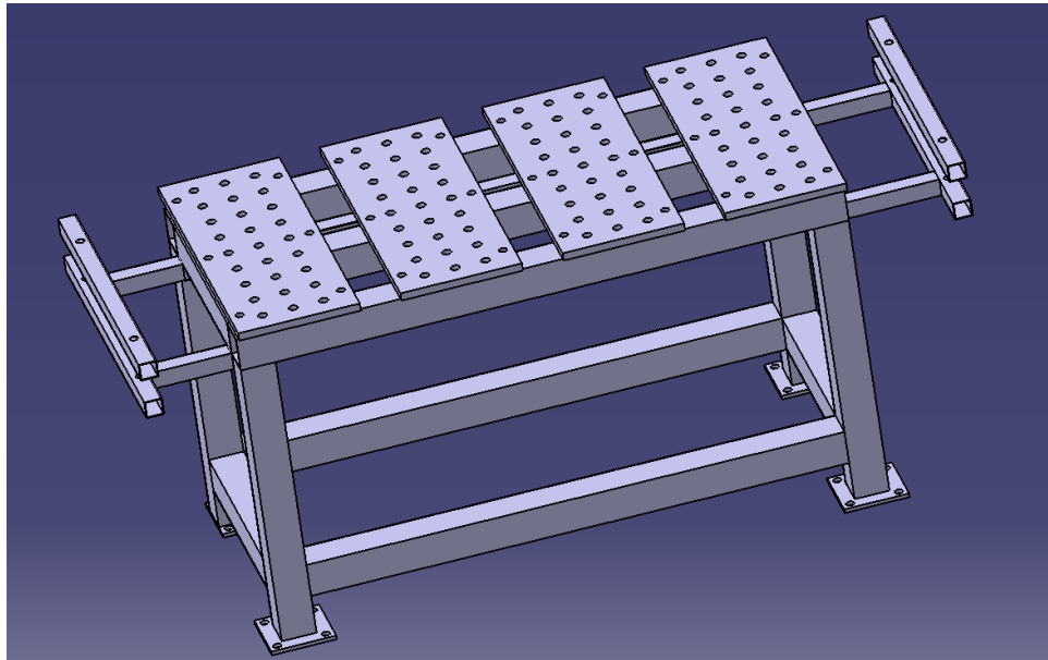
Abbildung 3.1: 3D-Modell des Schweißtisches im Gesamtzusammenbau
