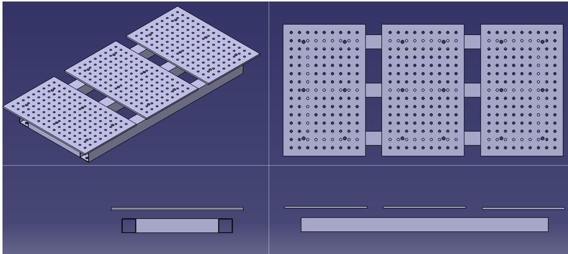
CAD-Ansicht von drei D16-Lochplatten 800×500×12 mm nebeneinander auf dem Schweißtisch-Rahmen – Isometrie, Draufsicht und Seitenansichten.
