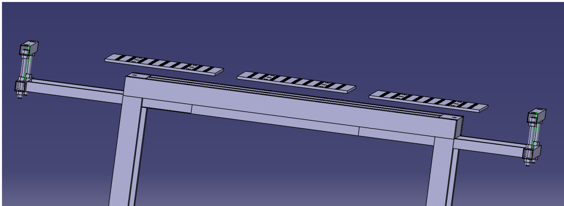
CAD-Darstellung des Teleskop-Erweiterungssystems: Führungsrohr mit Klemmschrauben und drei Auflageleisten mit Höhenverstellung.
