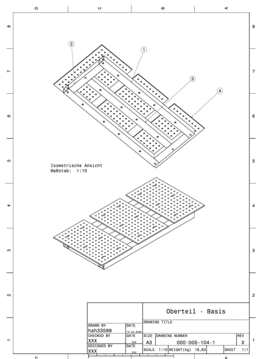
Oberteil-Basis 000-005-104-1 vom 10.04.2026: isometrische Ansicht mit drei Lochplatten auf Rahmen, Schriftfeld mit Gewicht 18,63 kg.
