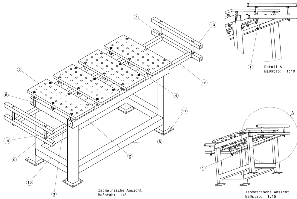
Isometrische Gesamtansicht mit Positionsnummern 1–14: Rahmen, Tischplatten, Auslegerarme, Fußplatten und Detailansicht der Verschraubung.
