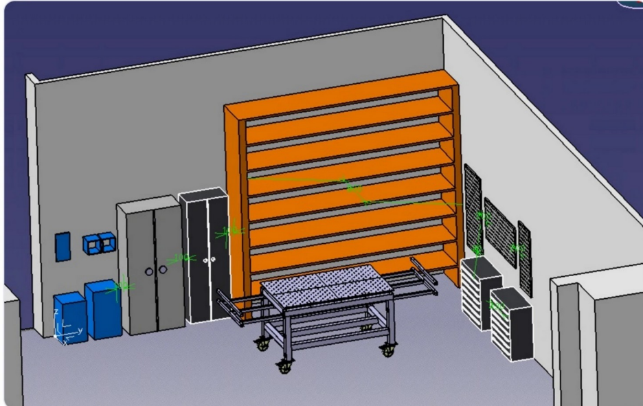
Abbildung 2.1: Ecke mit Materialregal (Mitte), Lochwänden (rechts), Schränken (links) und Schweißtisch
