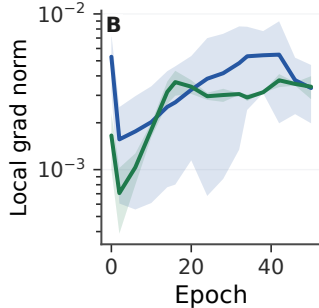
Local updates
