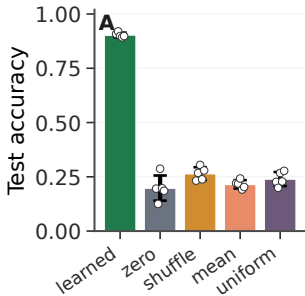
MNIST
