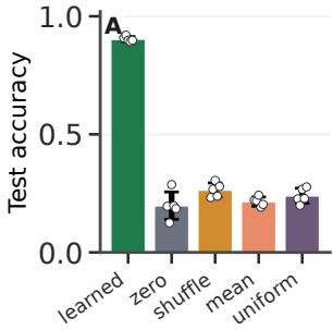
MNIST
