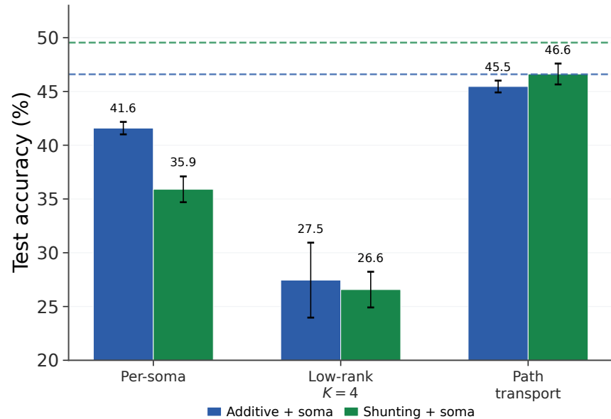
CIFAR-10 soma-on ladder
