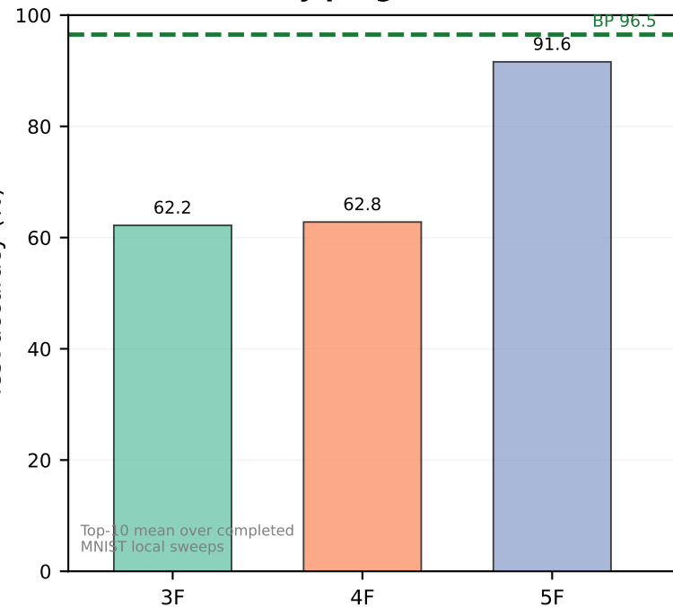
(D) Rule-family progression on MNIST
