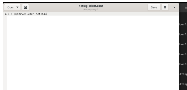
Figure 2: Настройка приёма записей журнала по TCP-порту 514.
