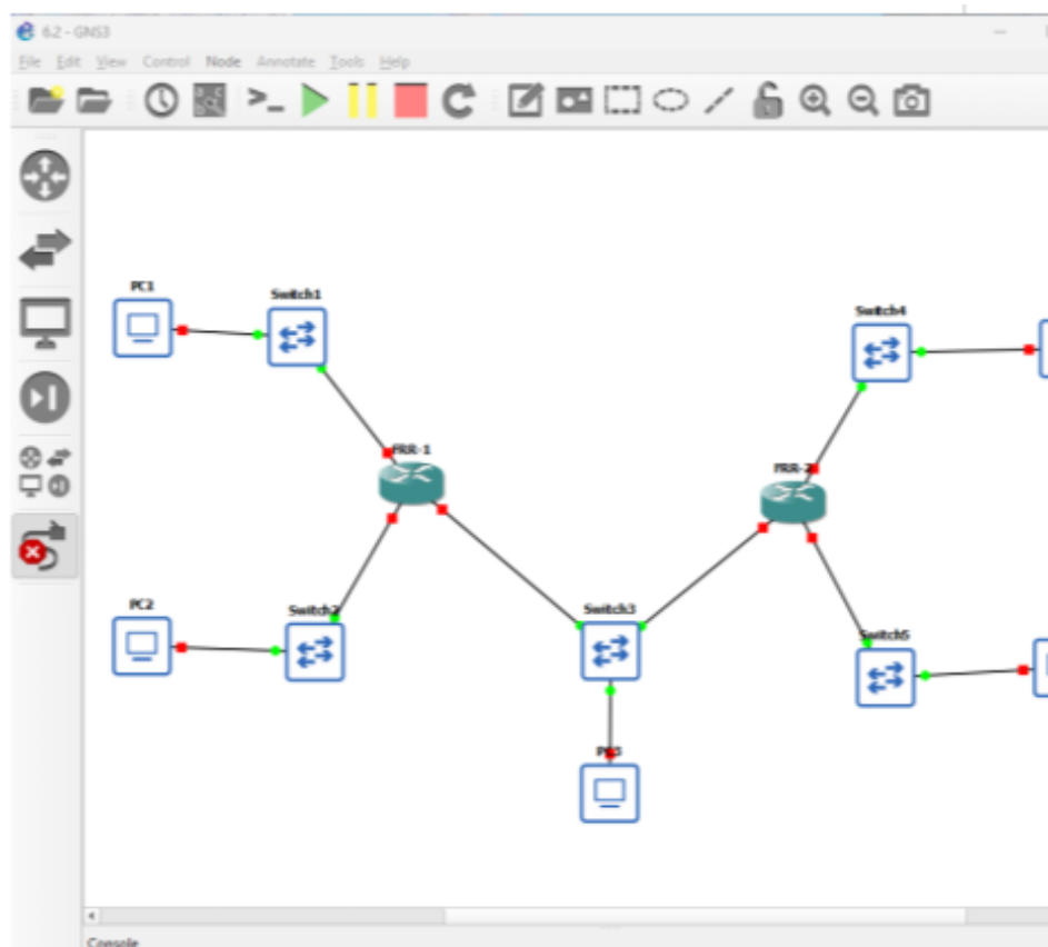
Рис. 6: Проверка состояния интерфейсов маршрутизатора
