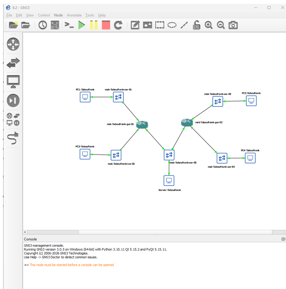
Рис. 16: Проверка изоляции IPv4 и IPv6 подсетей
