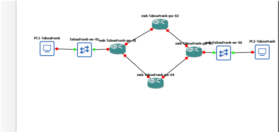
Рис. 1: Топология сети в GNS3
