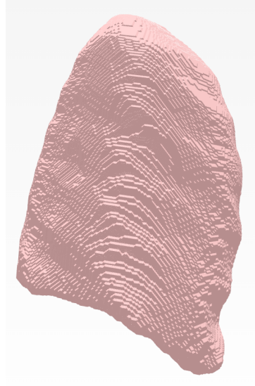
FIGURE 4.11 – Maillage avec faces colorées avant lissage : l’effet d’escalier lié à la discrétisation voxel est clairement visible sur le flanc du volume.
