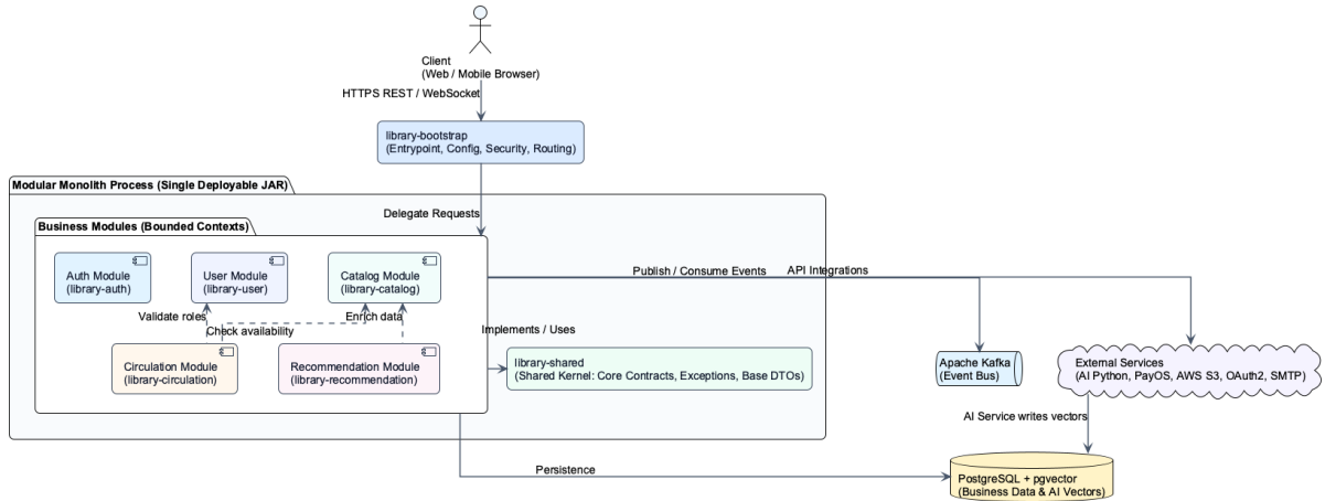
Hình 6.9: Sơ đồ kiến trúc Modular Monolith tổng thể
