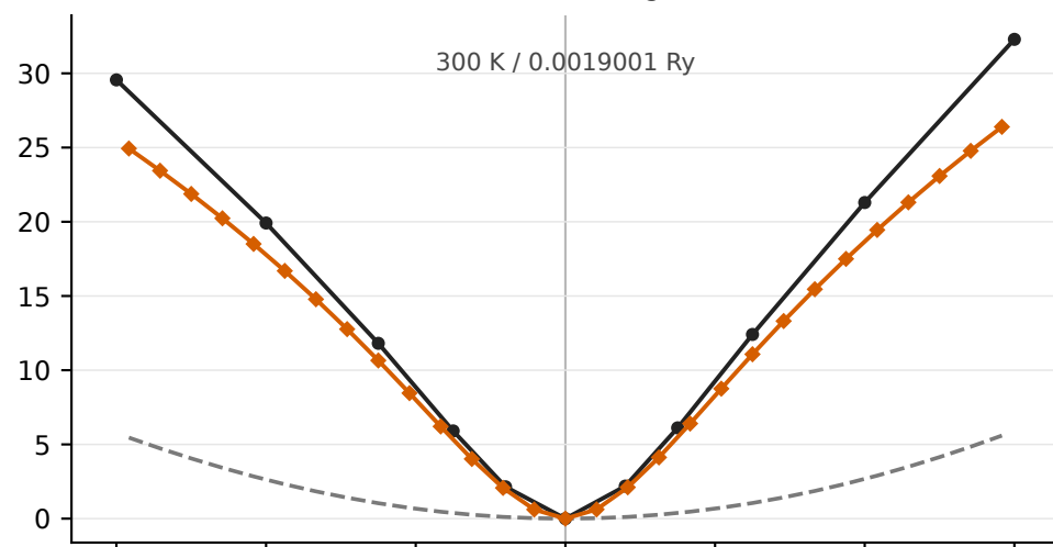
Quantum SSCHA background (Q0)
