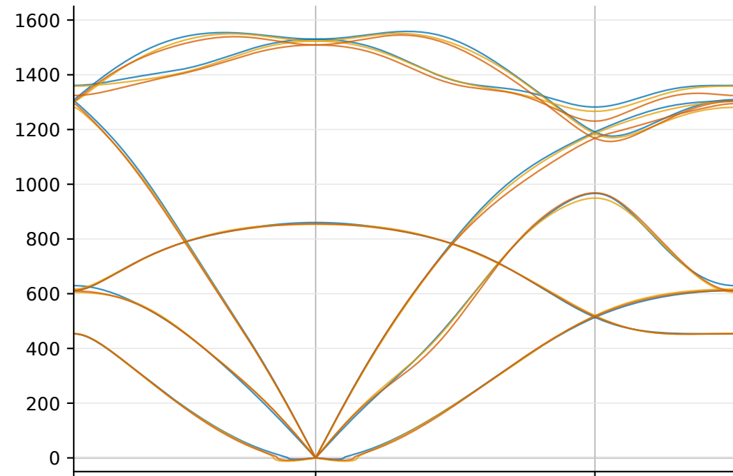
(b) Quantum SSCHA (Q0)
