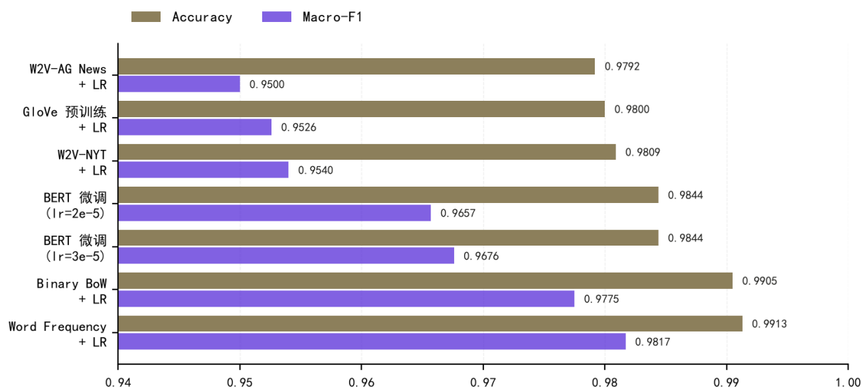
图 1 七组实验的 Test Accuracy 与 Macro-F1 对比
