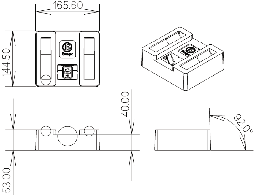
165.6*144.5*높이 53
