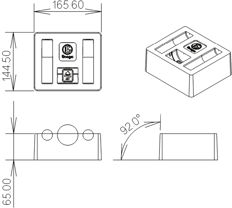
165.6*144.5*높이 65
