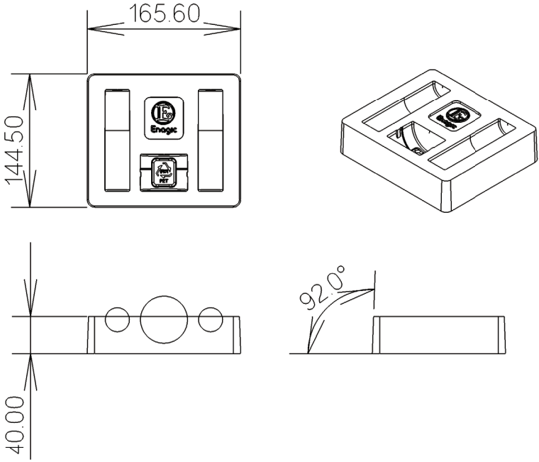
165.6*144.5*높이 40
