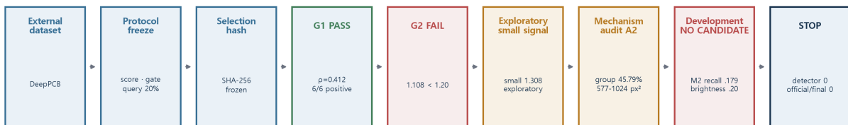
그림 4. DeepPCB prospective STOP case. 외부 protocol freeze부터 parent primary FAIL, exploratory signal의 분리 감사, development NO_CANDIDATE와 detector/official-test STOP까지의 authorization chain을 보인다. 이는 selector 성공 사례나 predictive accuracy가 아니라 process conformance 사례다.
