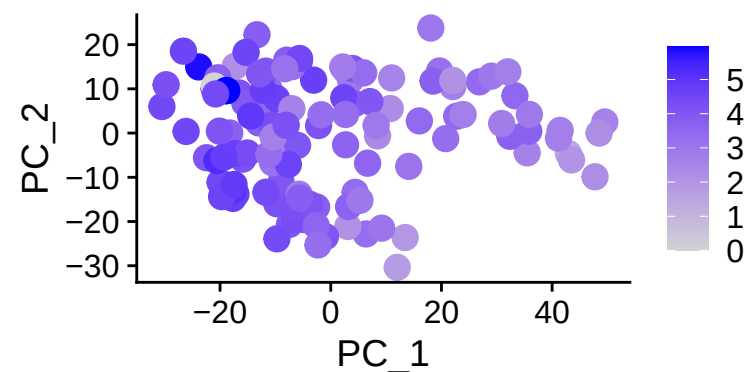
EGFL7
