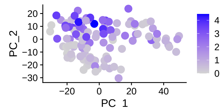
FMO2
