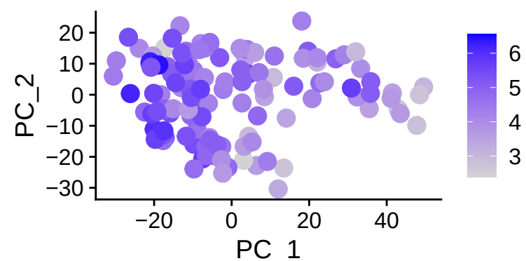
EGLN3
