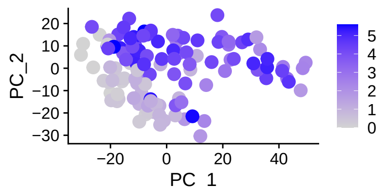
PDPN
