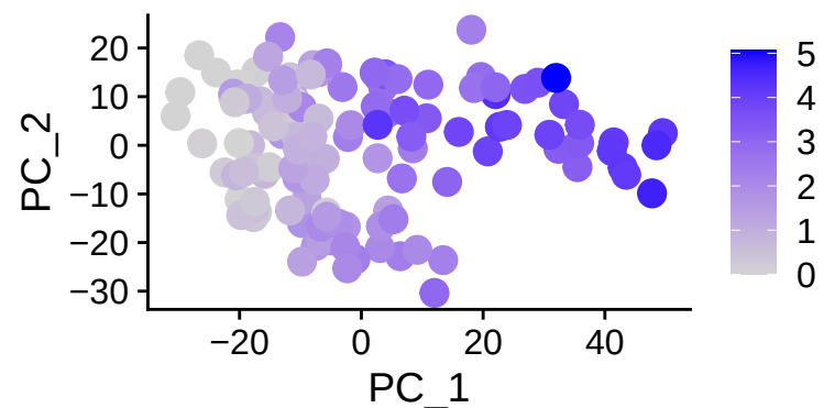
CXorf36
