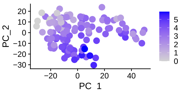
DMD
