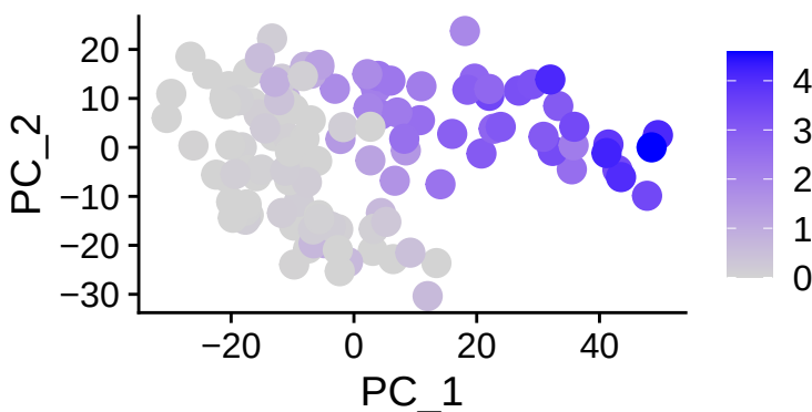
NES
