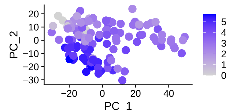
NOSTRIN
