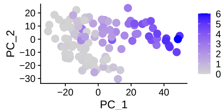
TSPAN18
