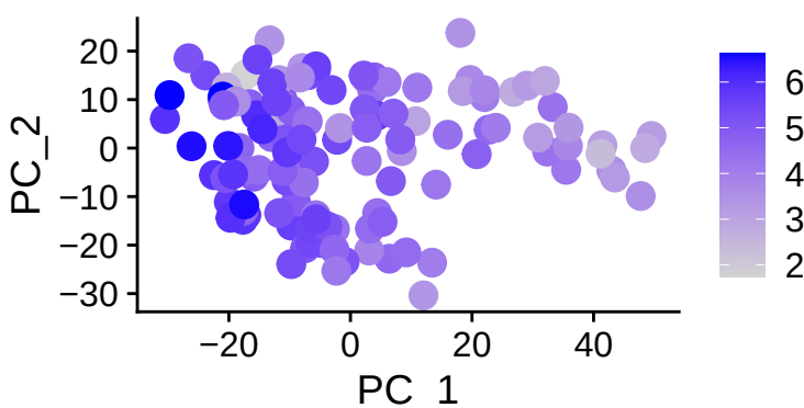
GPR1
