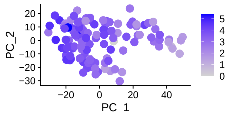
PROX1
