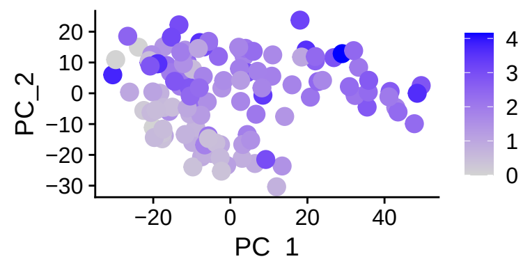
NEDD9
