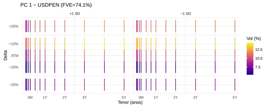
Figura 2: Primera eigensuperficie FPCA para USD/PEN.
