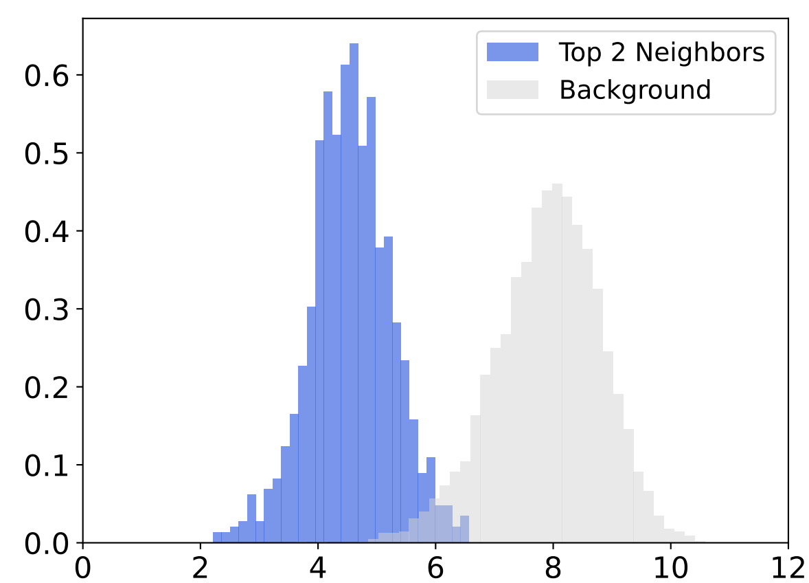
CLIP Latent Manifold (K=2)
