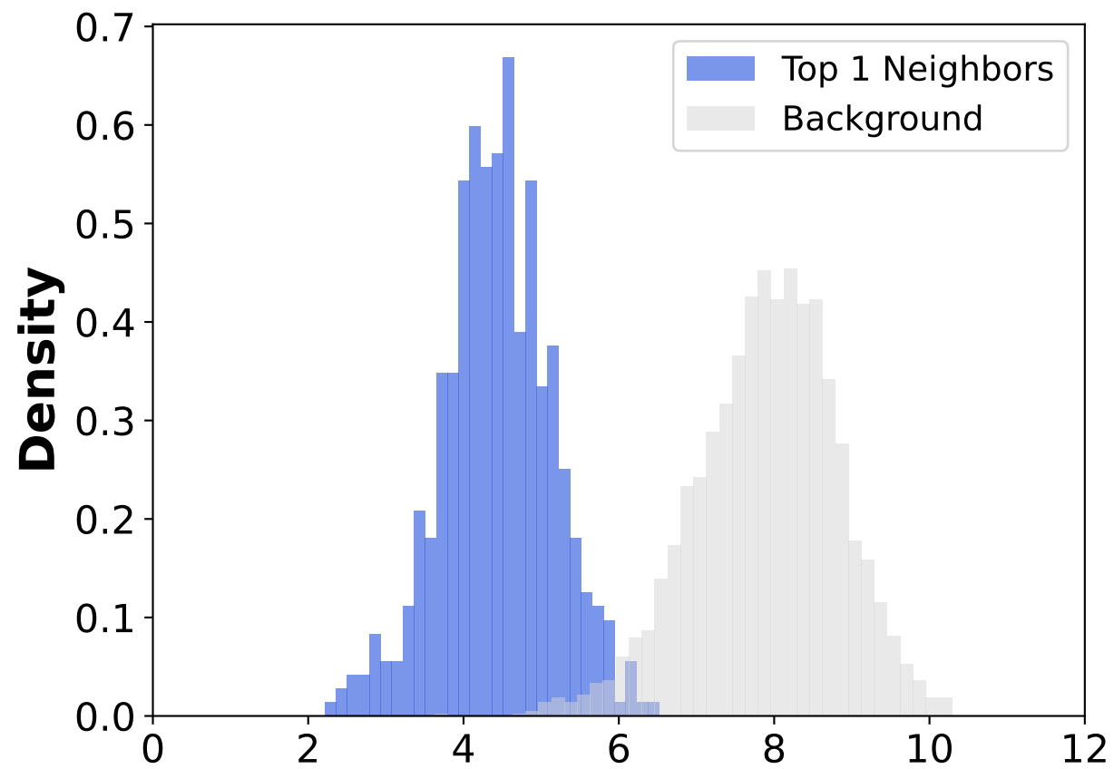
CLIP Latent Manifold (K=1)
