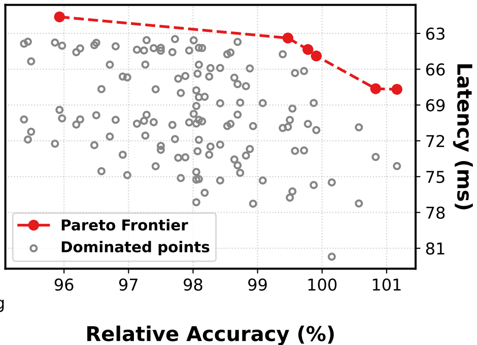
Pareto Frontier
