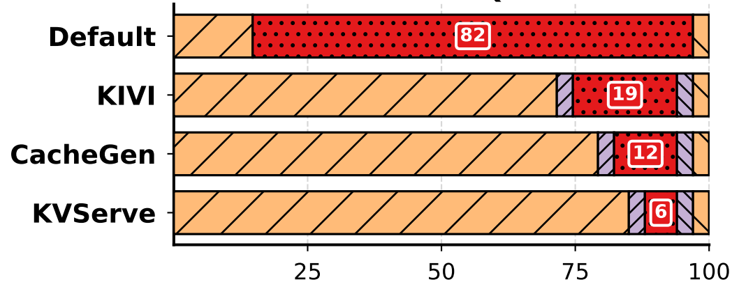
2WikiMQA
