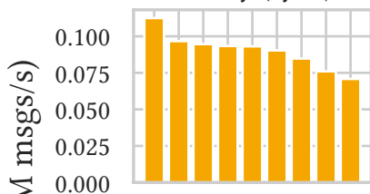
NATS (sync)
