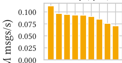
NATS (sync)
