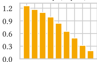
NATS (async)
