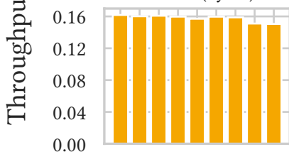
Pulsar (sync)
