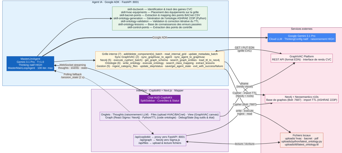
Figure 3 – Architecture finale de SI-Mapper — un agent maître unique avec des compétences spécialisées, des outils et une interface de visualisation.
