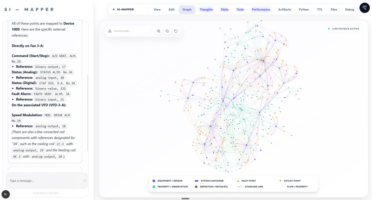
Figure 10 – Système 3 : vue complète du graphe sémantique ASHRAE 223P dans la visualisation Neo4j de SI-Mapper.
