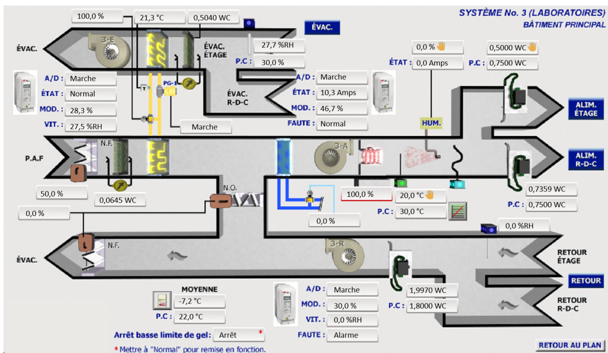
Figure 8 – Système 3 : plan d'ingénierie HVAC original utilisé comme entrée pour l'agent.
