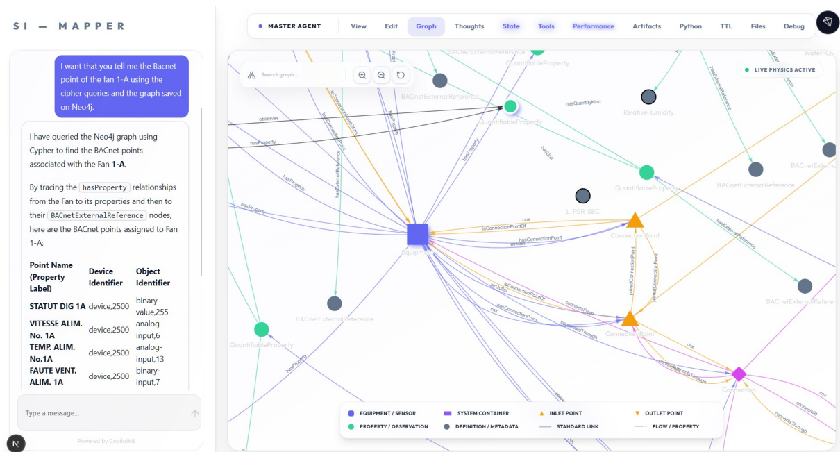
Figure 7 – Système 1 : vue détaillée de la topologie des équipements, montrant les nœuds avec leurs points de connexion et les références externes BACnet.
