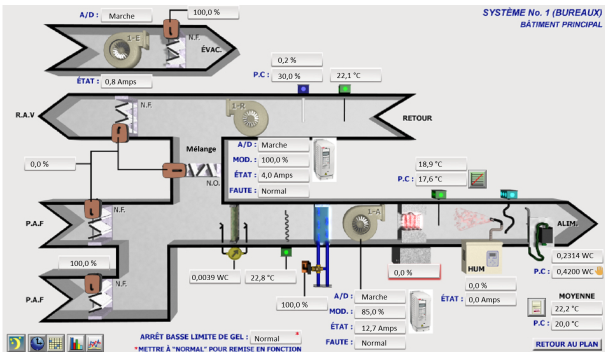
Figure 4 – Système 1 : plan d'ingénierie HVAC original utilisé comme entrée pour l'agent.
