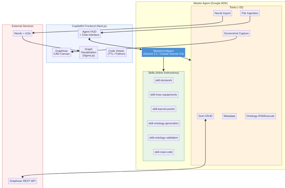
Figure 3 – Architecture finale de SI-Mapper — un agent maître unique avec des compétences spécialisées, des outils et une interface de visualisation.
