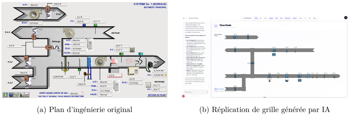
Figure 4 – Système 1 : schéma HVAC original (gauche) et la réplcation de l'agent sur la grille Graphivac (droite), produite comme étape intermédiaire avant la génération ASHRAE 223P.
