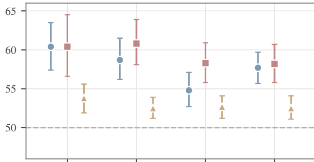
(d) InternVL3-8B: modal answer share
