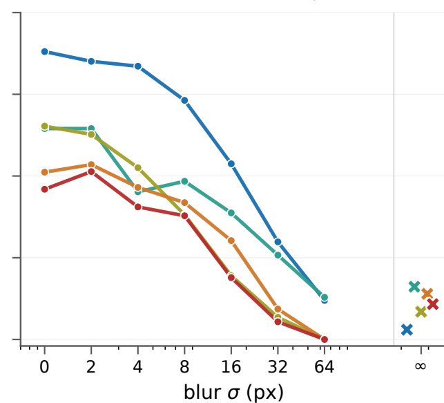
Claude Sonnet 4.6
