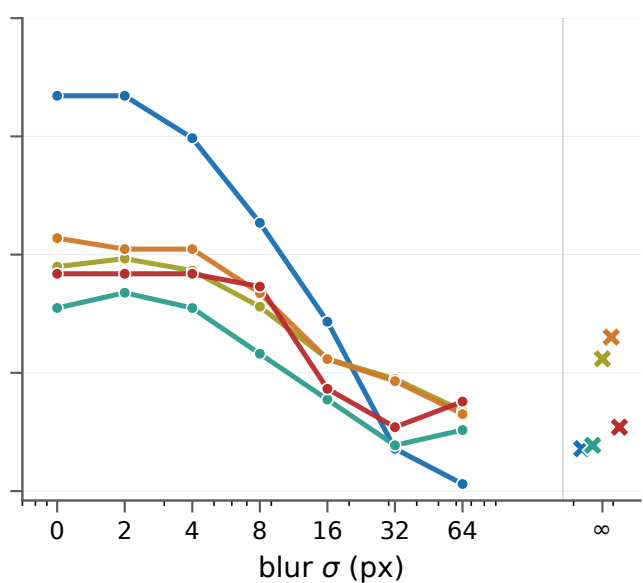
HuatuogPT-V 7B
