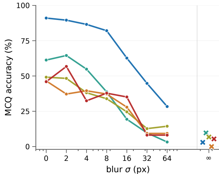
GPT-4o
