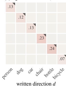
(e) Qwen3-VL-32B, COCO
