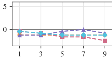
MedXpertQA
