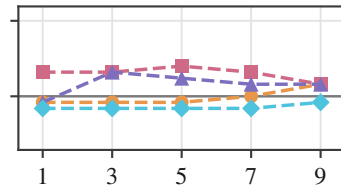
MedQA (USMLE)
