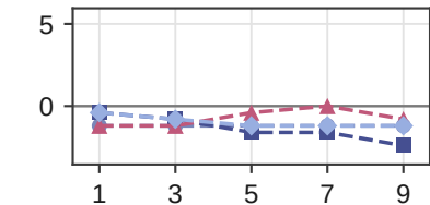
MedXpertQA
