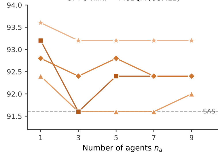
GPT-5 mini · MedQA (USMLE)
