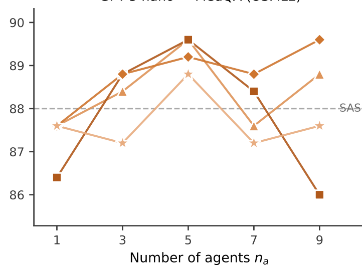
GPT-5 nano · MedQA (USMLE)
