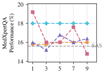
GPT-4.1 nano
