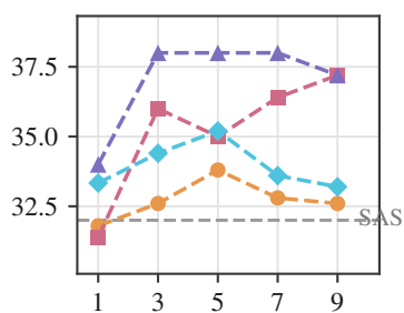
GPT-5 nano
