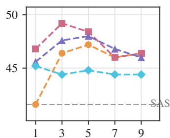
GPT-5 mini
