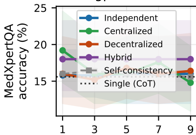
T1 gpt-4.1-nano
