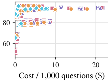
MedQA (USMLE)
