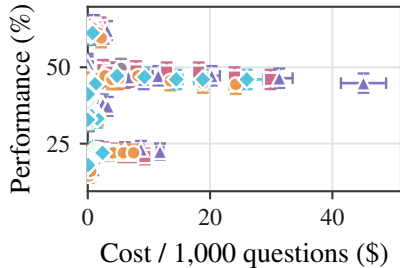
MedXpertQA
