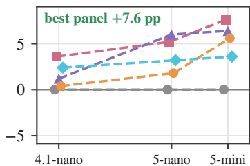
MedXpertQA
