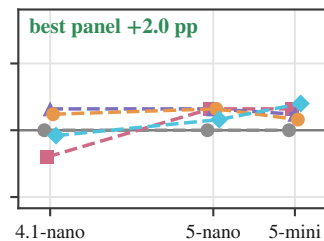
MedQA (USMLE)
