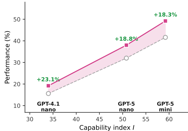
MedXpertQA
