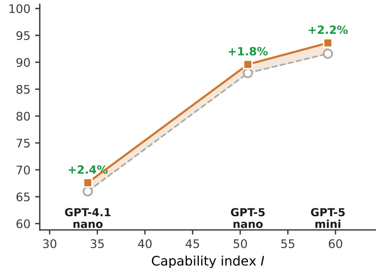
MedQA (USMLE)
