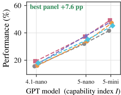
MedXpertQA
