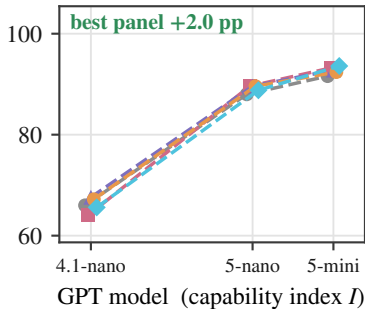
MedQA (USMLE)
