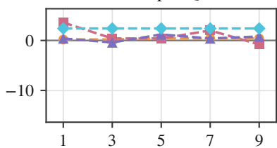
MedXpertQA
