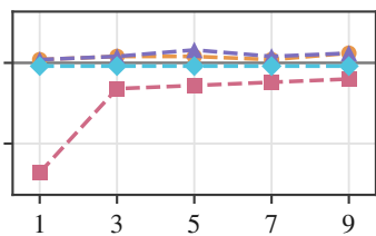
MedQA (USMLE)
