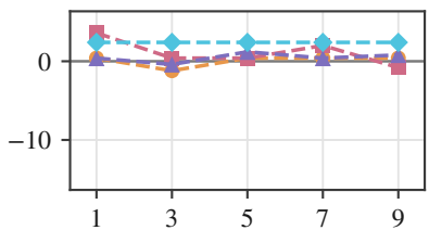
MedXpertQA
